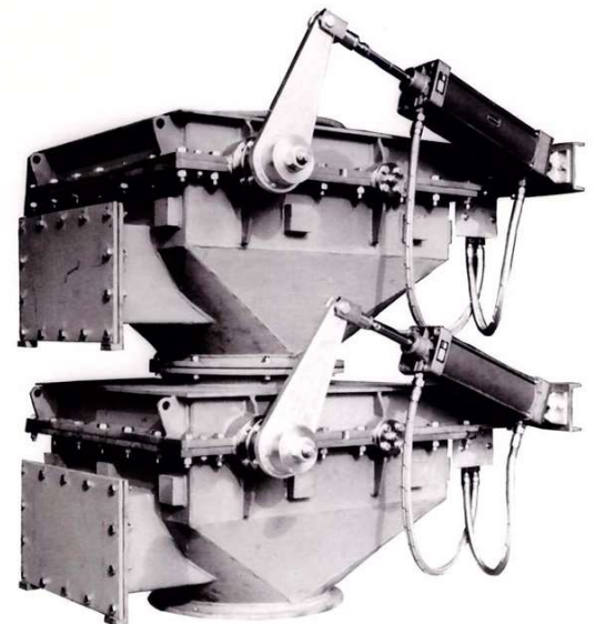
Bild 5: Doppelklappenschleuse DKS500T
