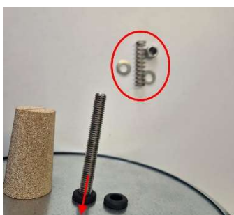
Freigemachter Bolzen steht jetzt frei in der Gummidurchführung des Deckels
